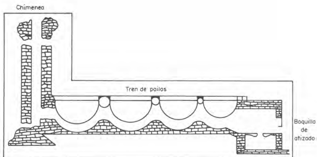
Fig 2 Vista lateral de un tren de 4 Pailas, Jamaiquino.
