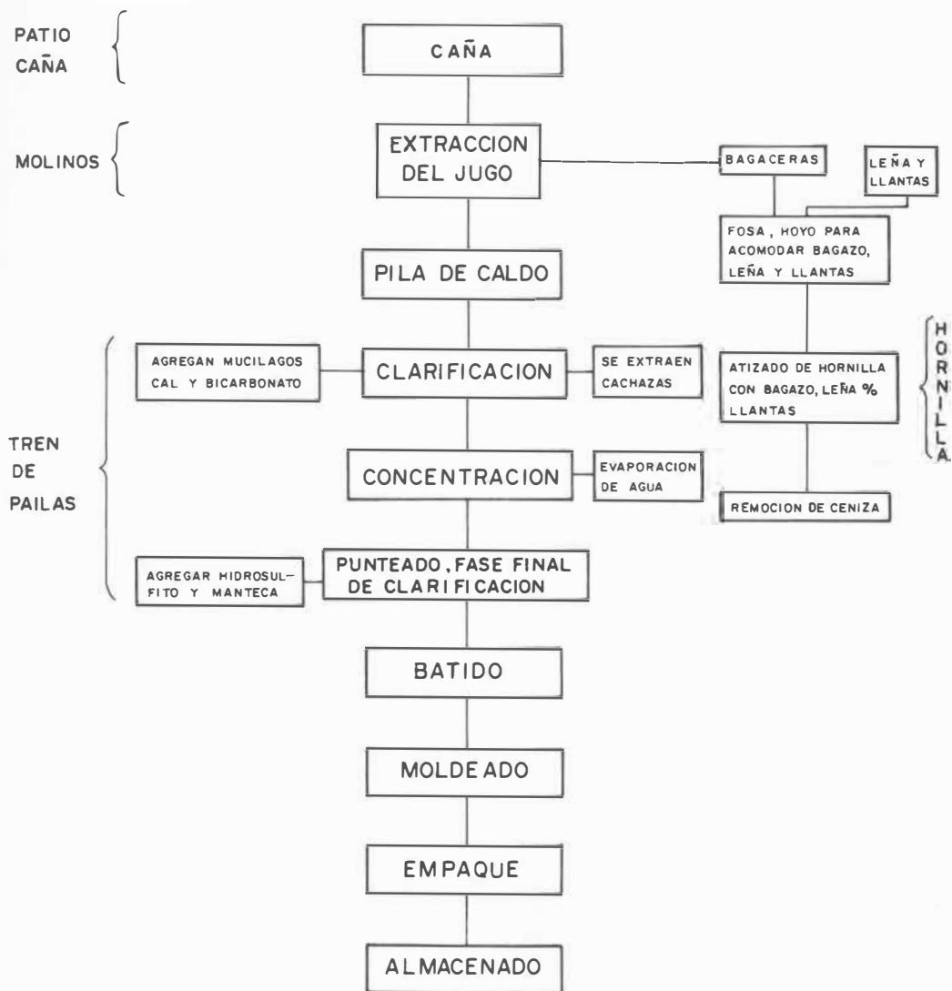
Fig. 1. Diagramo del proceso de fabricación de topo de dulce
